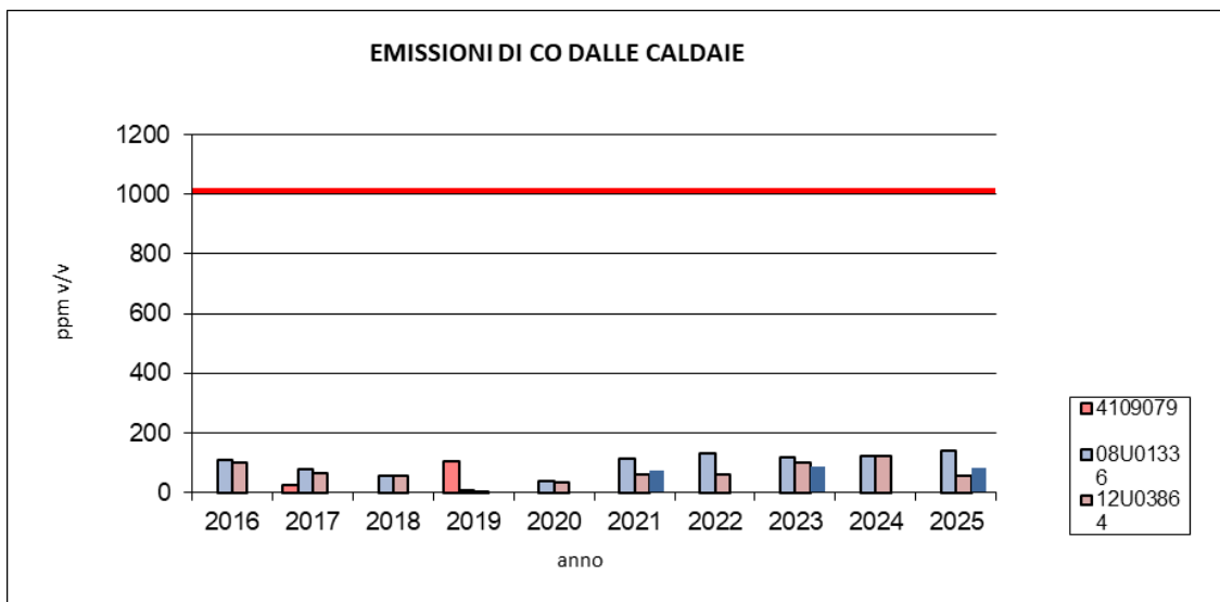
Fig.15 Andamento delle emissioni di CO (monossido di carbonio dalle caldaie)
