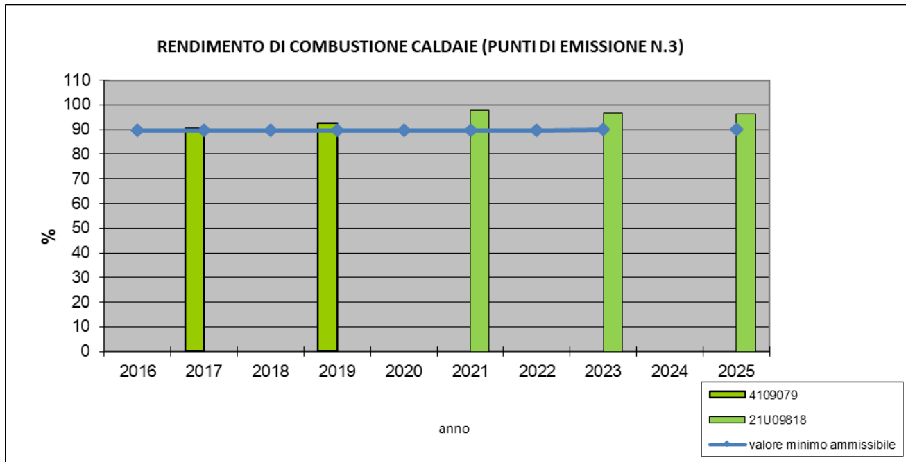
Figura. 14 Andamento del rendimento di combustione relativo al punto di emissione n. 3
