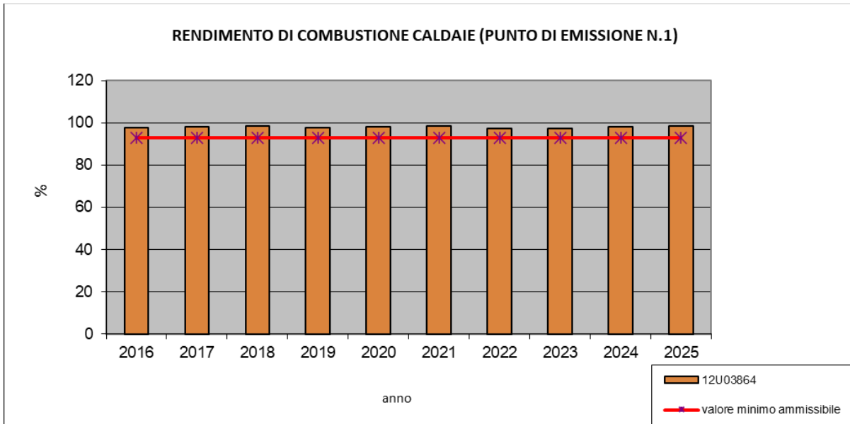
Fig. 12 Andamento del rendimento di combustione relativo al punto di emissione n. 1
